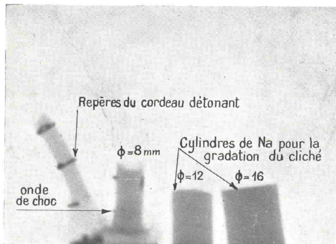
FIG. 15. — Radiographie d'une onde de choc dans le sodium correspondant à 17 000 kg/cm 2 .
